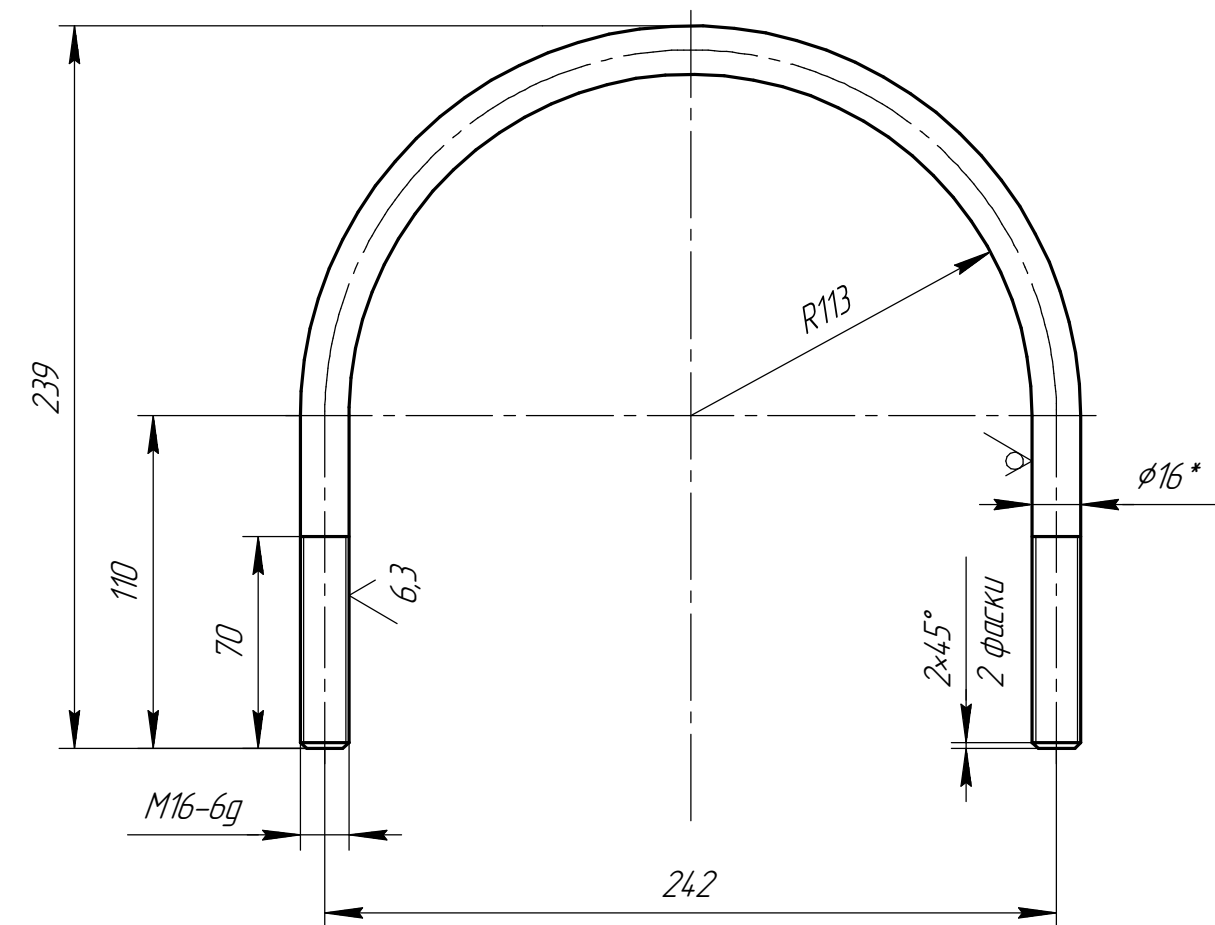
Дет. поз. 4
