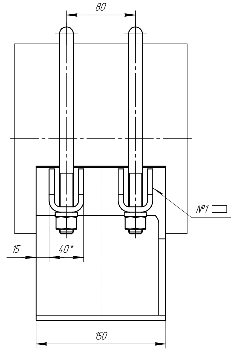
Дет. поз. 2
